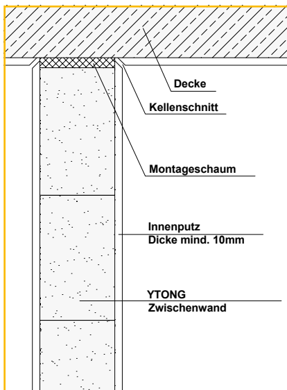
Gleitender Deckenanschluss
