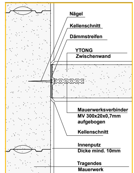
Gleitender Wandanschluss
