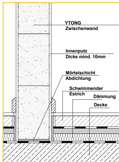
Gleitender Fußpunkt
