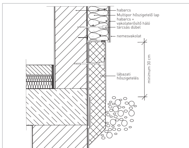
Lábazatkialakítás
